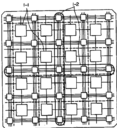
プログラマブル論理素子の構成
